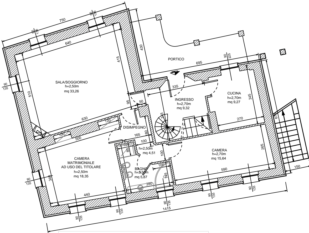
PIANTA PIANO TERRA/RIALZATO rapp. 1:100 PIANO ABITATIVO
